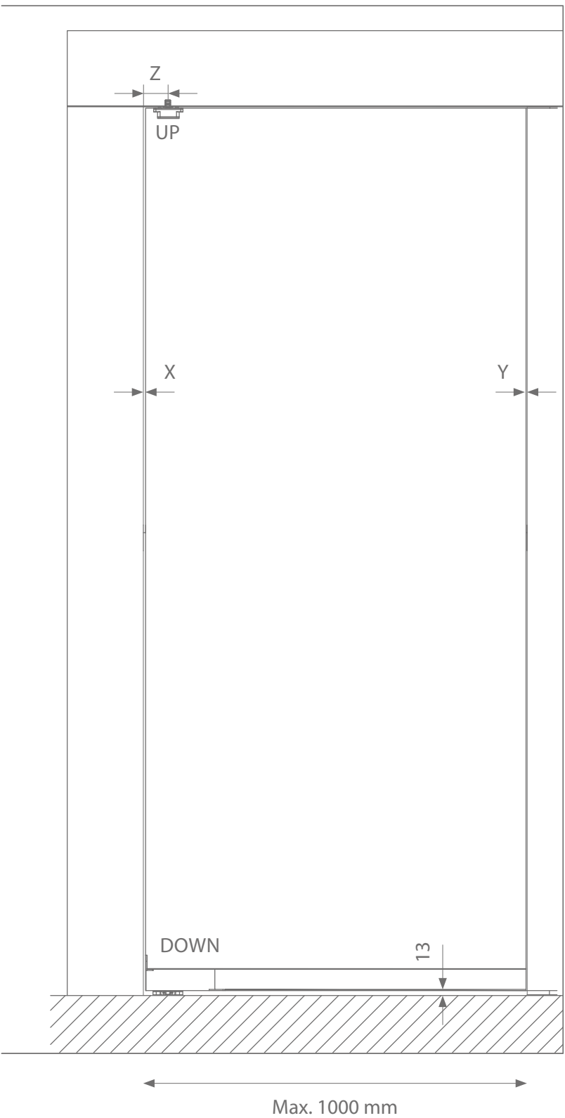
LINTEEL MONTAGE / MONTAGE SOUS LINTEAU / LINTEL MOUNT / MONTAGE IM STURZ / MONTAJE DINTEL
