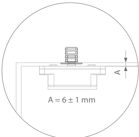
LINTEEL MONTAGE / MONTAGE SOUS LINTEAU / LINTEL MOUNT / MONTAGE IM STURZ / MONTAJE DINTEL
