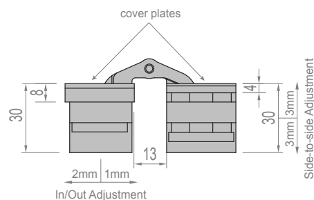
FRAME DOOR
